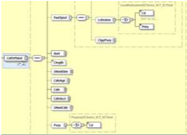
Abbildung 41: pain.001.001.09, Credit Transfer Transaction Information (Ausschnitt nur Delta SCT/SCTInst)
