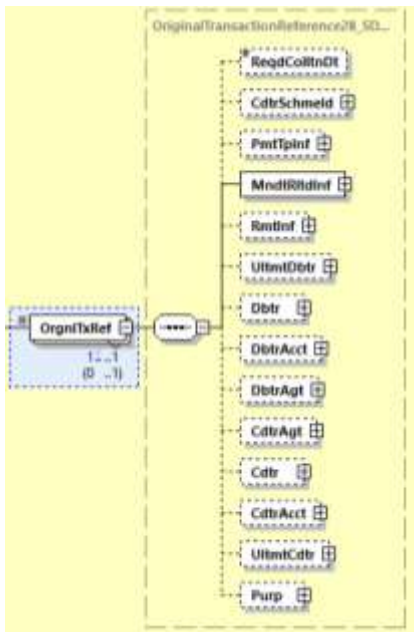
Abbildung 122: Übersicht pain.007.001.09, OrgnTxRef
