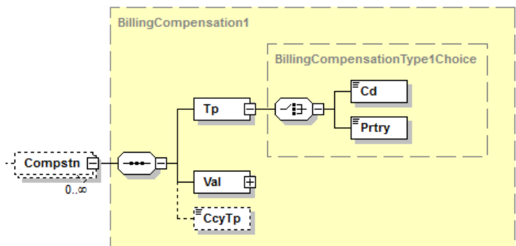
Abbildung 149: Übersicht camt.086.001.02, Compstn
