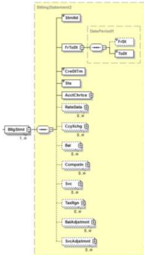
Abbildung 144: Übersicht camt.086.001.02, BlgStmt
