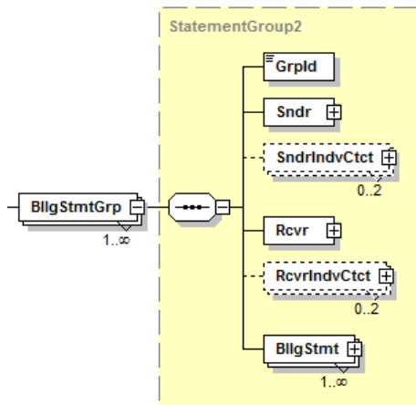
Abbildung 141: Übersicht camt.086.001.02, BllgStmntGrp
