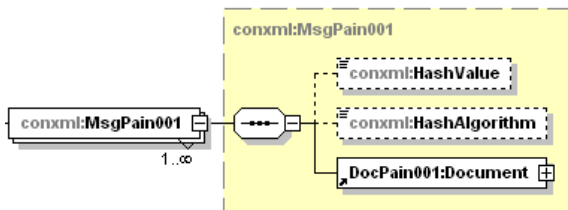
Abbildung 115: container.nnn.001.GBIC4, Message (beispielhafte Auswahl)
