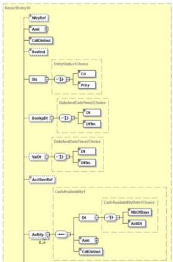
Abbildung 85: camt.053.001.08, Ntry (Fortsetzung Folgeseite)
