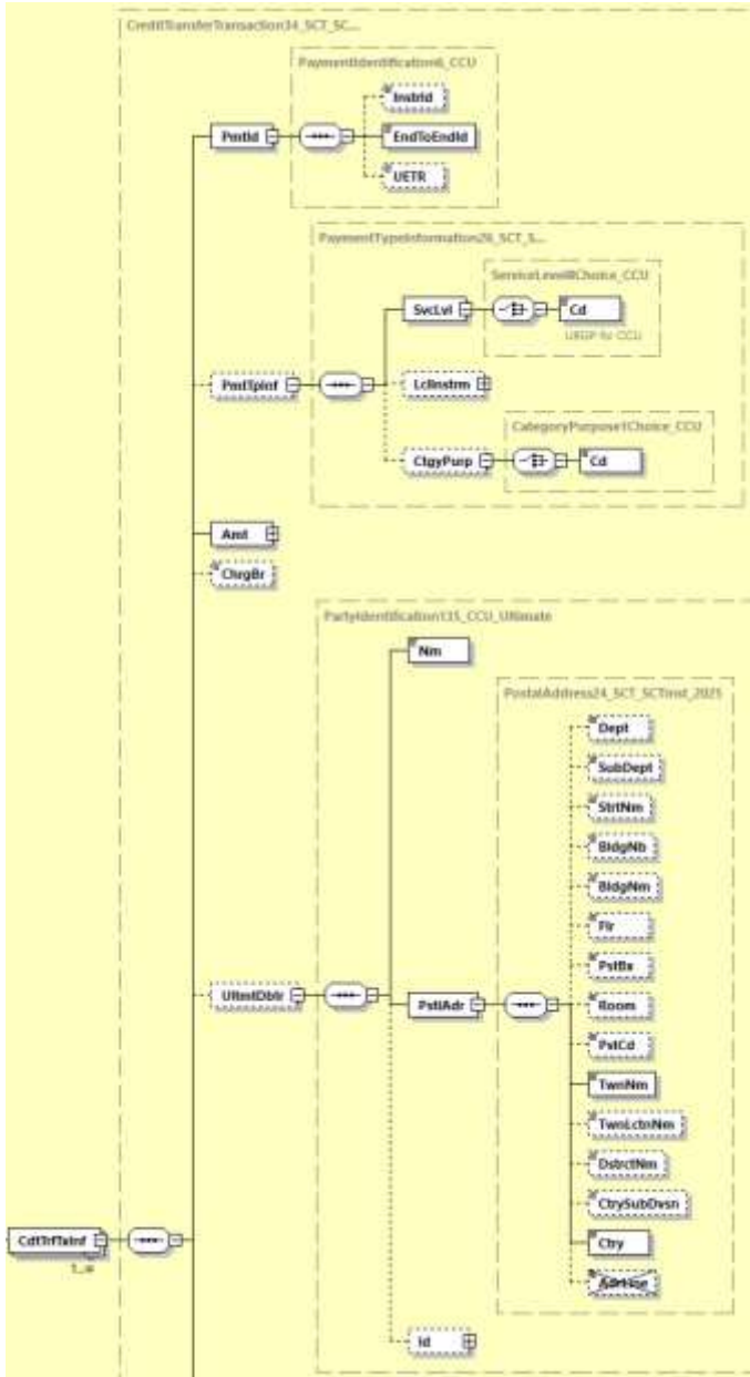
Abbildung 117: pain.001.001.09, CreditTransferTransaction (Delta zu SEPA-Überweisung) – Teil 1
